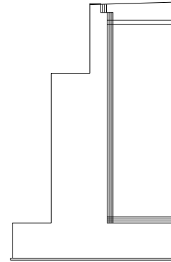
날개벽(우측)
