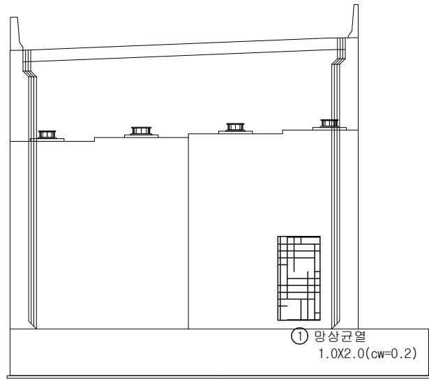
정면도
