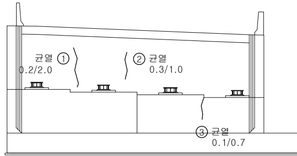
정면도
